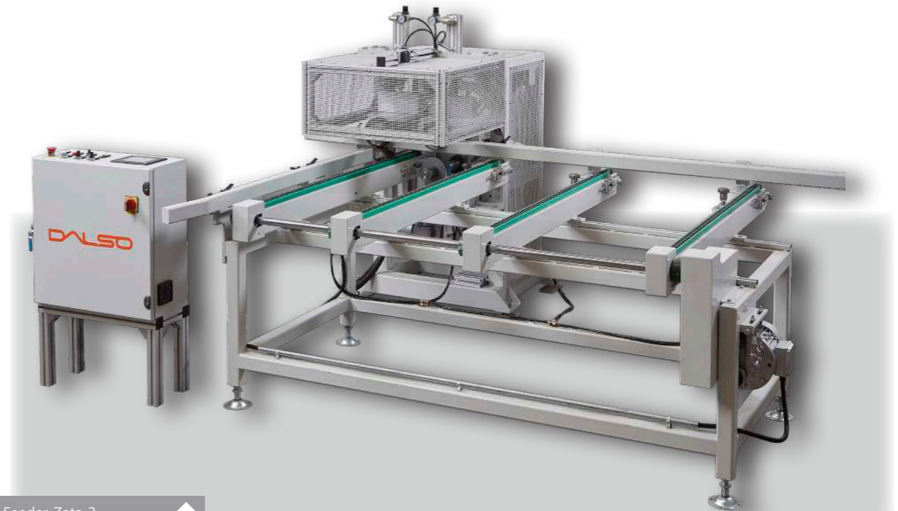
Feeder Zeta 2 Introduttore Zeta 2
